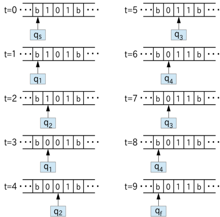
図2 チューリング機械の動作例
