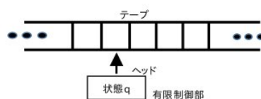
図 3.1: チューリング機械の概要
